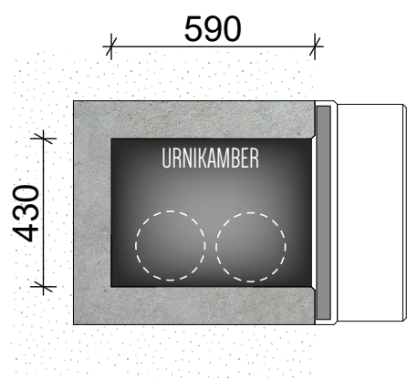
URNIKAMBER PLAAN
