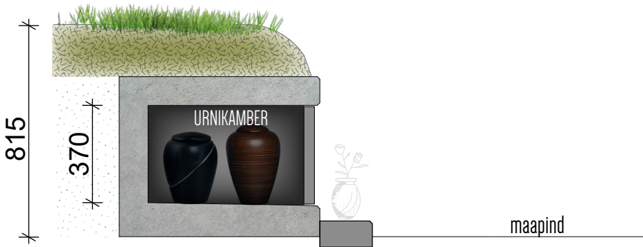
MADAL URNIMÜÜR LÕIGE
