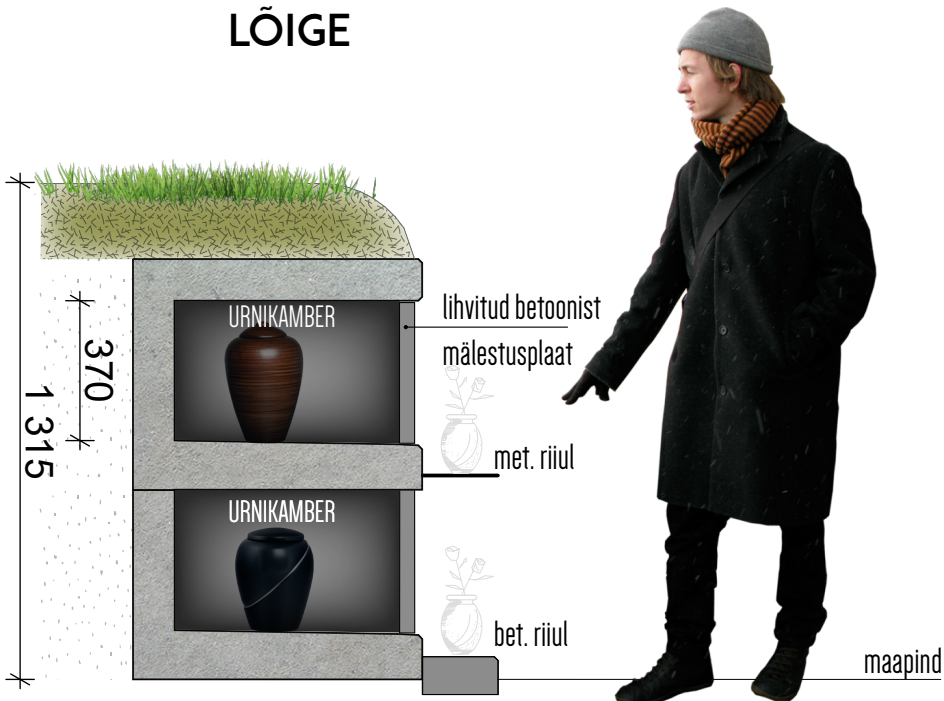
KÕRGEM URNIMÜÜR LÕIGE
