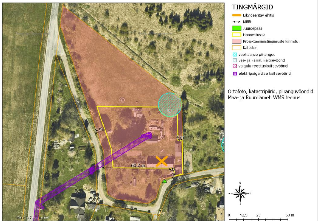
Joonis 1. Hoonestusala skeem
